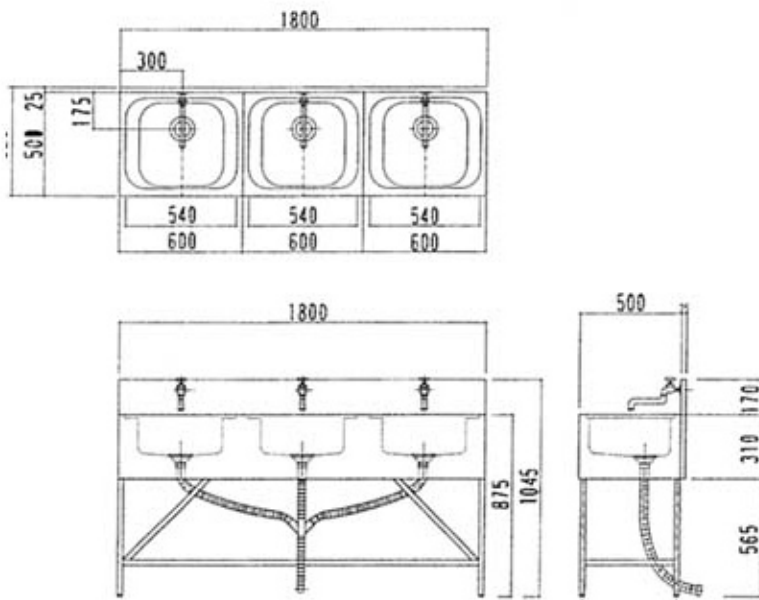
三槽シンク (HC-3 型) W1800×D525×H1045
