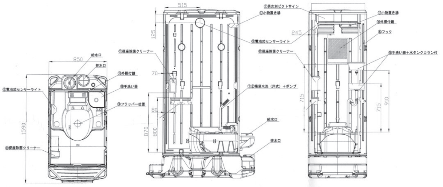
平面図
