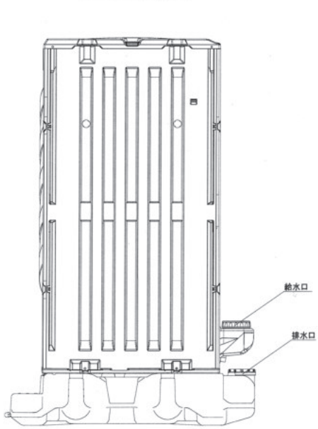
B 立面図
