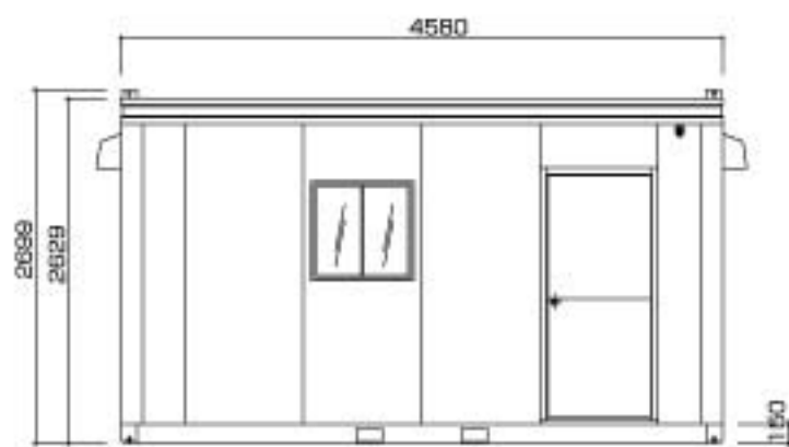
正面図
